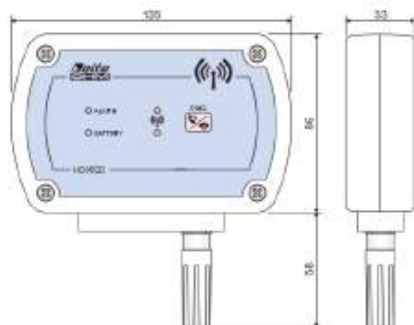
HD35ED... versiones con sonda HR+T fija
