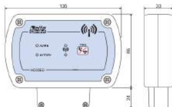
HD35ED... versiones con abrazaderas
