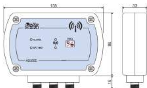
desde 1 a 3 conectores en función del modelo HD35ED... versiones con conectores M12
