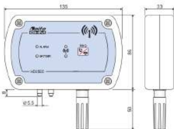
HD35ED... versiones con conexiones para presión diferencial (con y sin sonda HR+T fija)
