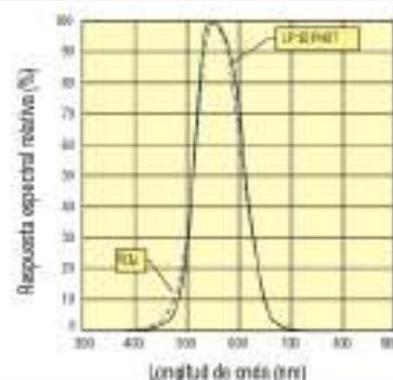
Gráfico 1 – Respuesta espectral relativa del sensor de iluminancia
