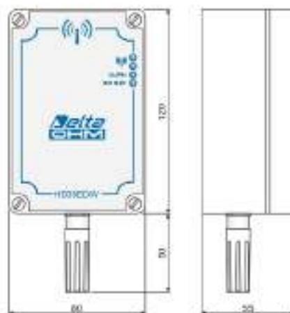
HD35EDW... versiones con sonda HR+T fija
