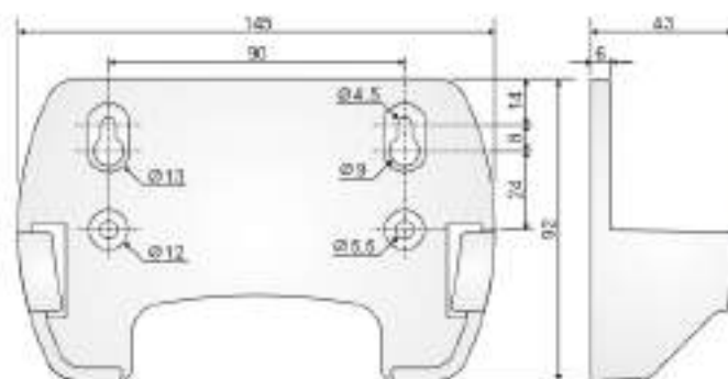
Soporte para instalación desmontable
