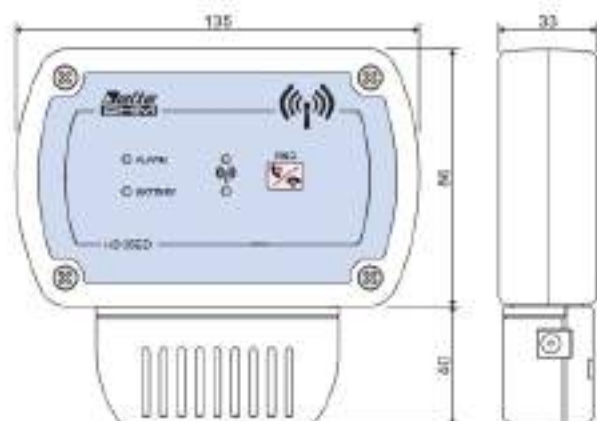
HD35ED... versiones con grilla
