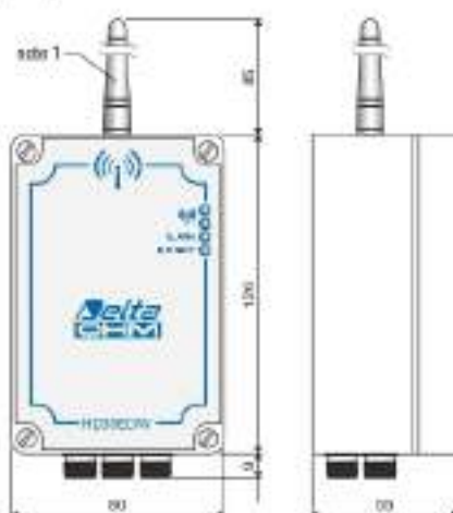
HD35EDW... versiones con conectores M12
