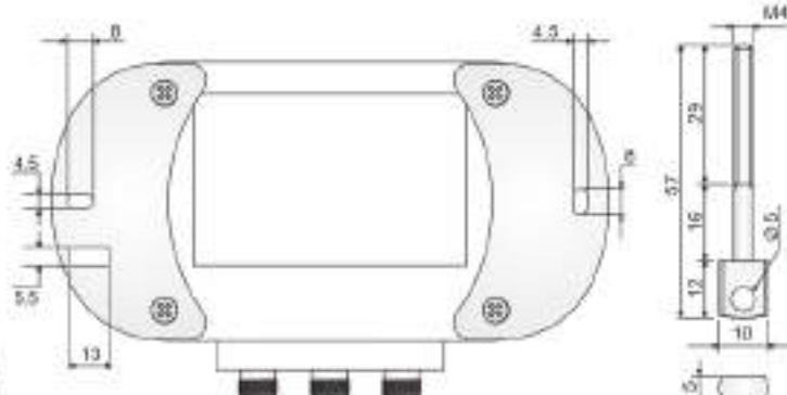
Bridas para la instalación fija
